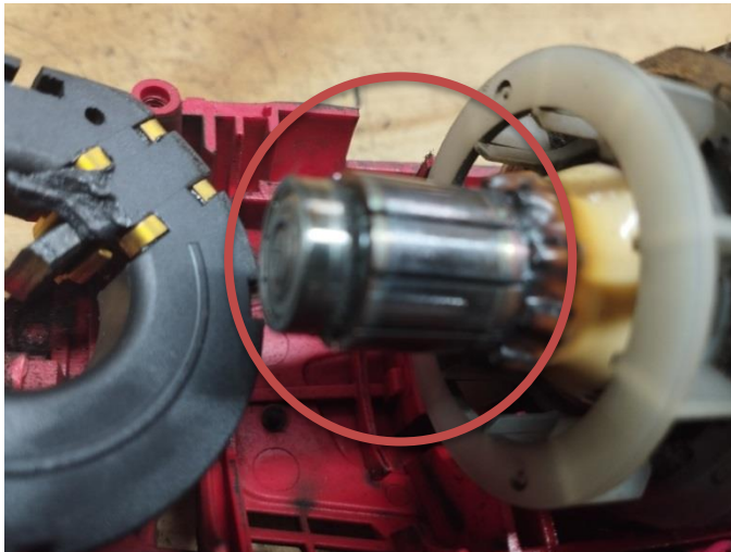
Obr. 2 Poškodenie komutátora
